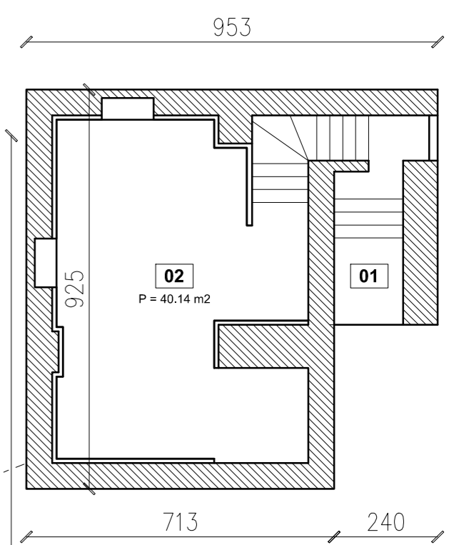
ОСНОВА ПОДРУМА
