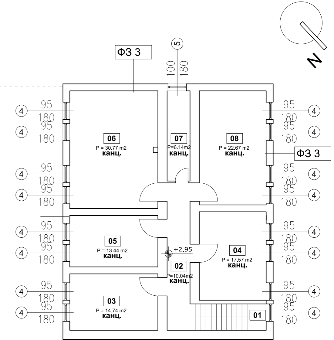
ОСНОВА МЕЋУСПРАТА
